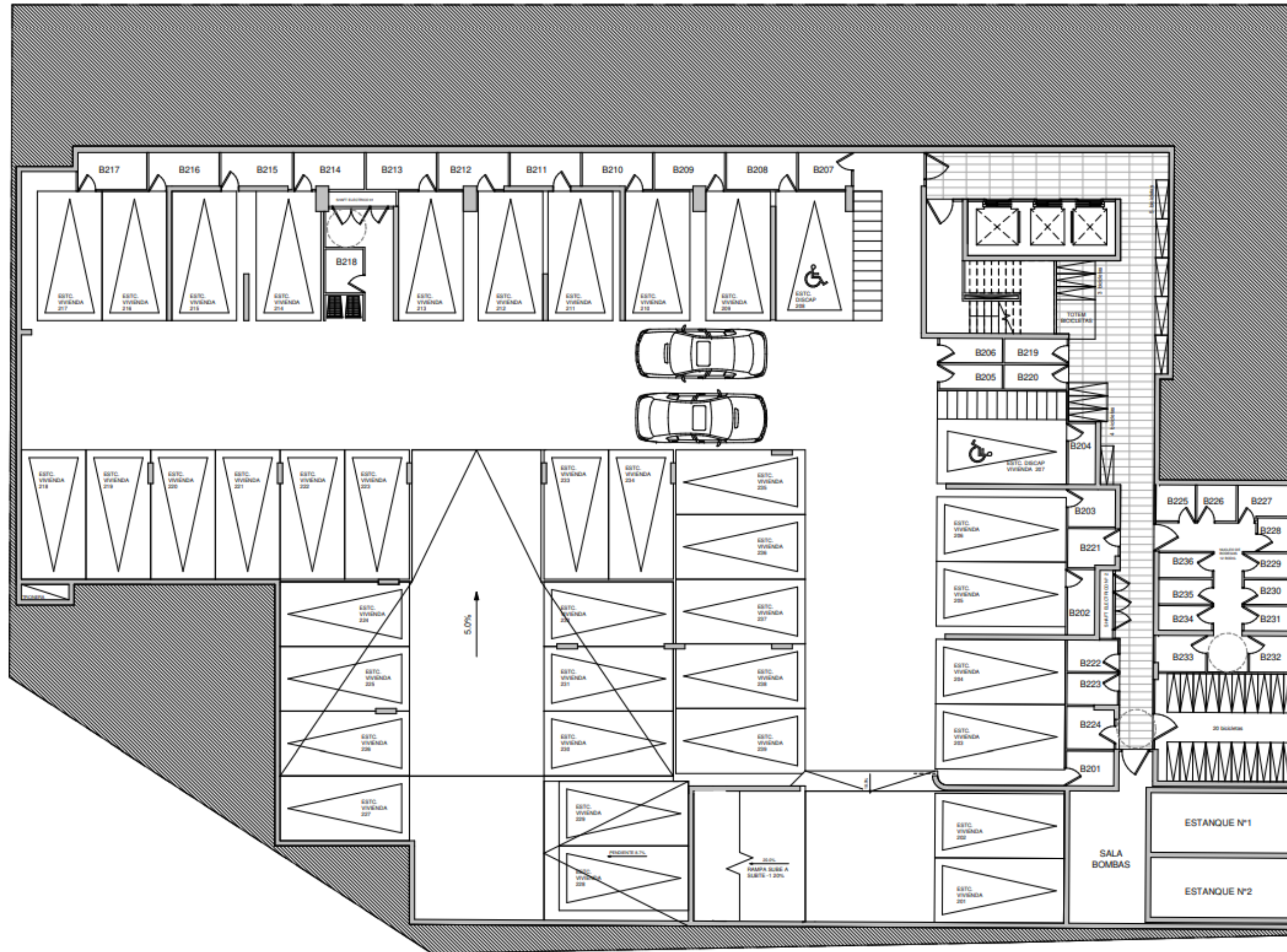
1 SUBTERRANEO -2 1 : 100
