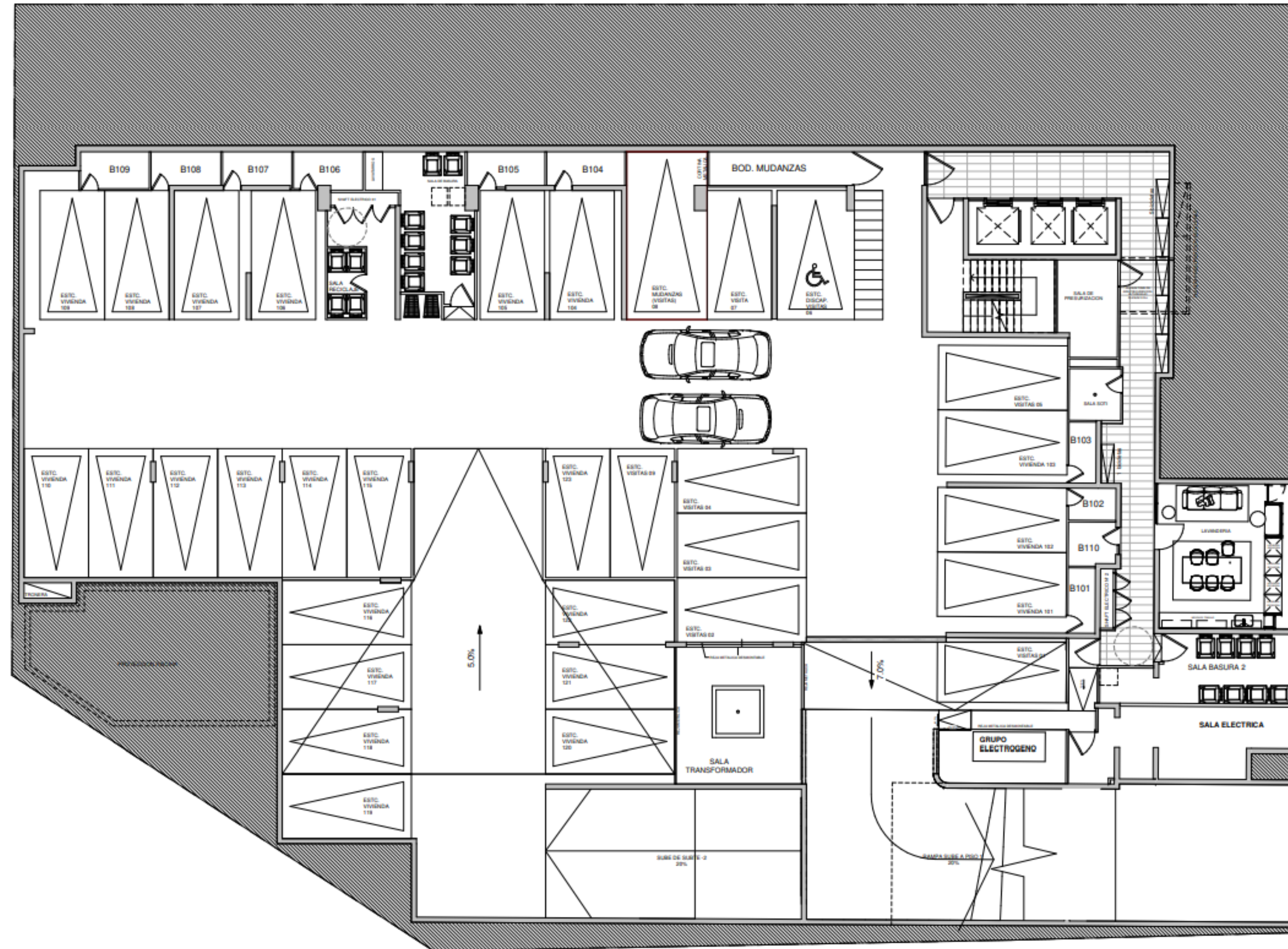
1 SUBTERRANEO -1 1 : 100
