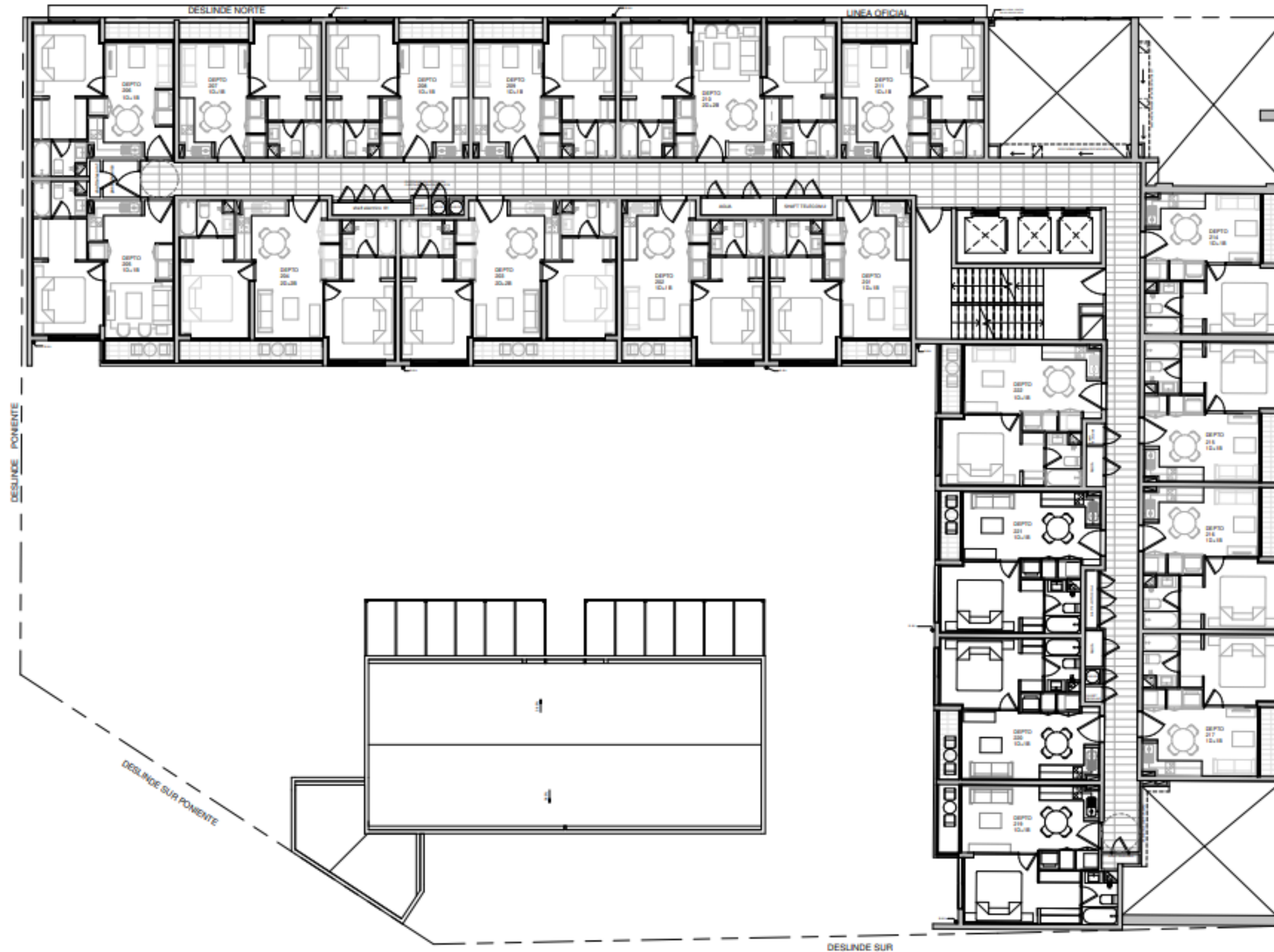
1 PISO 2 1:100
